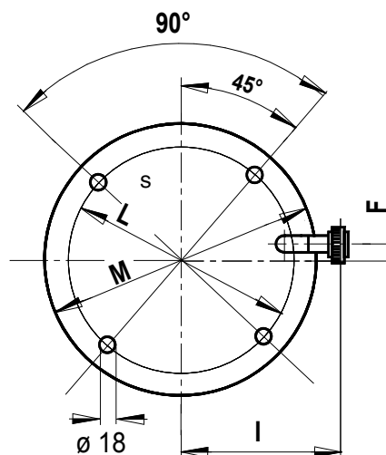
Размеры 32 / 40-125
