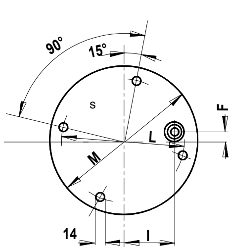
Размеры 15 -25
