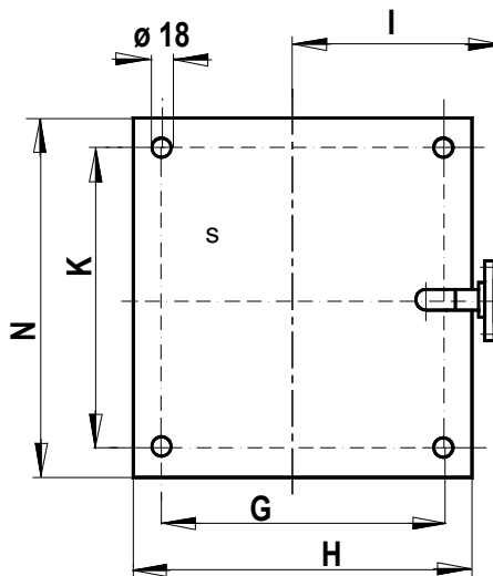
Размеры 65 - 80
